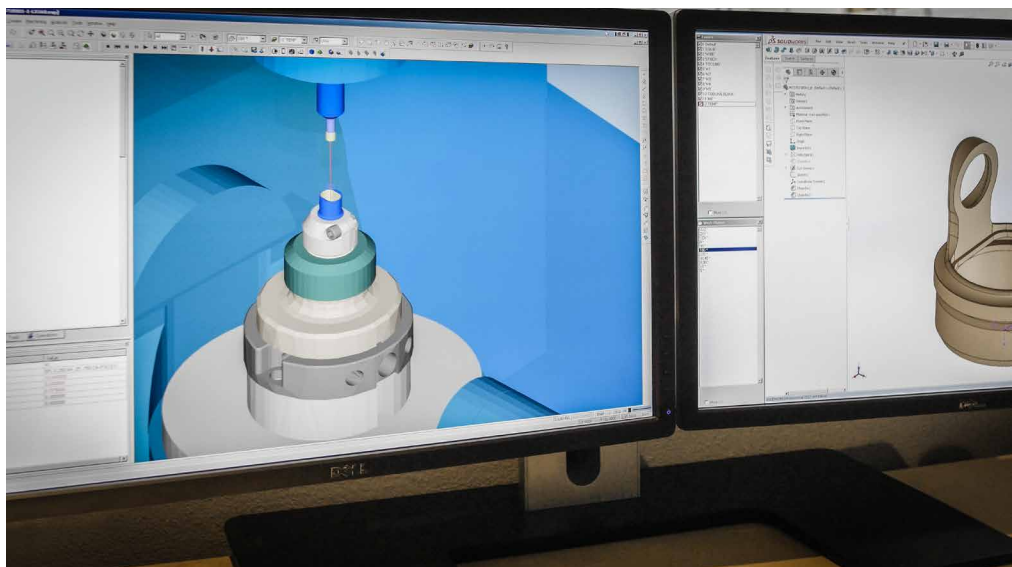
➤ Симуляция ESPRIT для проверки фрезерной / токарной детали перед началом производства
