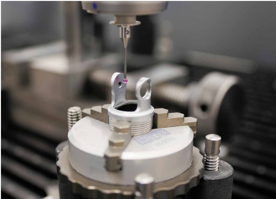
🔴 CMM проверка готовой детали, запрограммированной в ESPRIT
