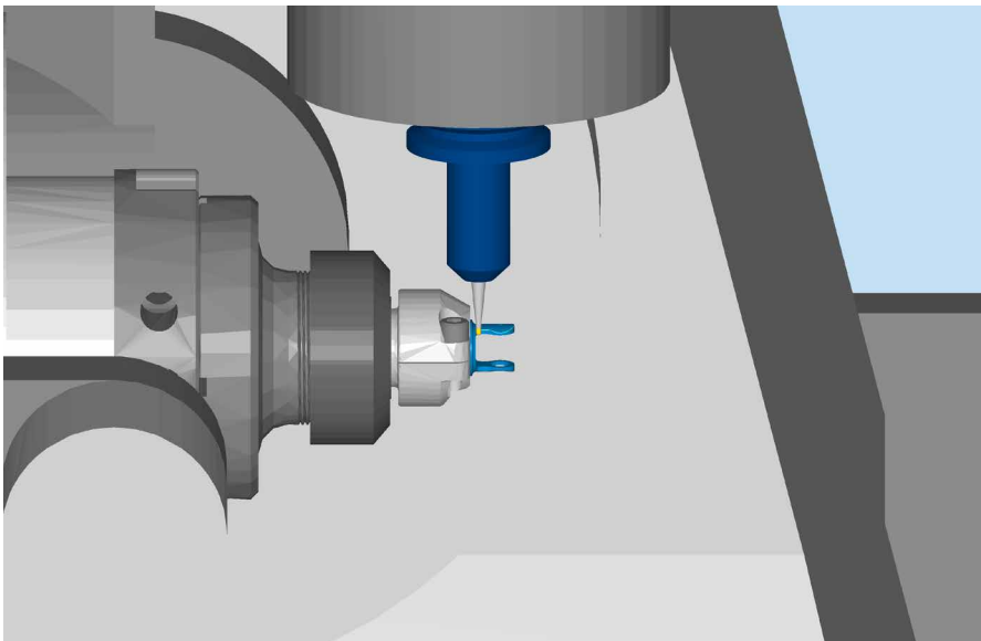
🔴 Симуляция ESPRIT для проверки фрезерной / токарной детали перед началом производства
